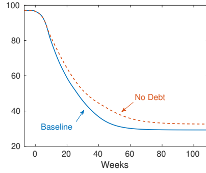
(d) Susceptible
