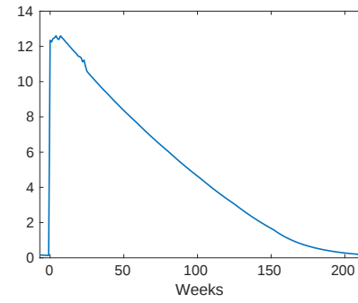
(d) Spread
